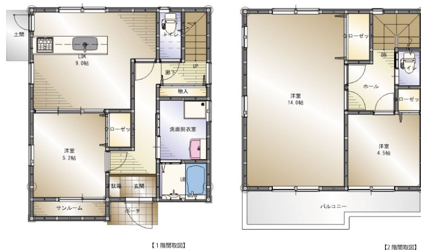
【間取り図】
