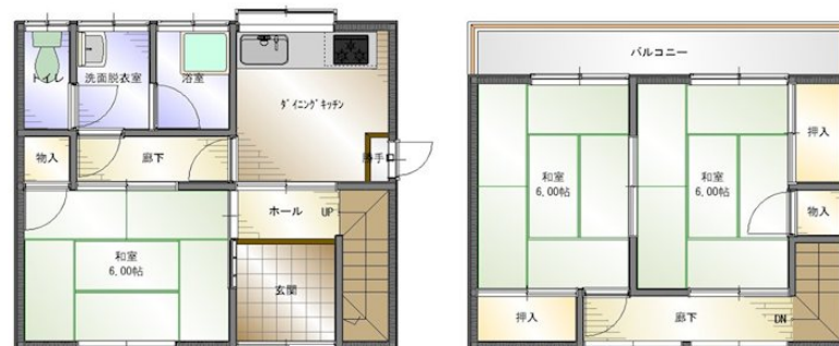
【1階 間取り図】
