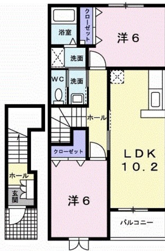
【間取り図】
